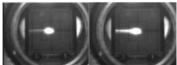
(a) エネルギー広がり小 (b) エネルギー広がり大 図1: スクリーンモニタによるエネルギー広がり測定
