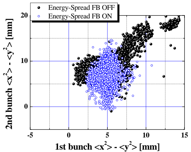
図5：アーク部ESMによるエネルギー広がりフィードバックの結果(10nCモード、1パンチ目のフィードバック目標値を5に設定した場合)
