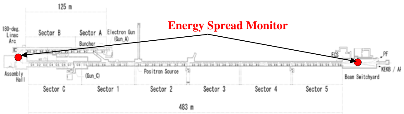
図2：KEK入射器のレイアウト及びエネルギー広がりモニタ設置場所
