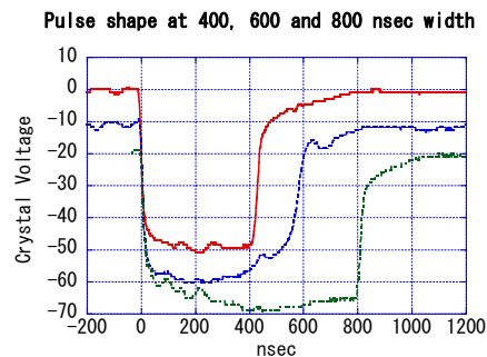
図4：400, 600, 800nsの代表パルス波形
