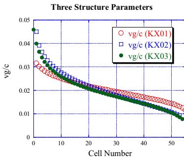
図1：60cm管パラメータ
