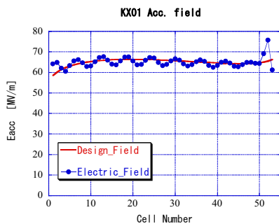
図2：KX01加速管の電界
