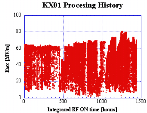
図3：KX01プロセッシング履歴
