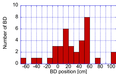
図6：最終長期ラン(>65MV/m)での放電分布
