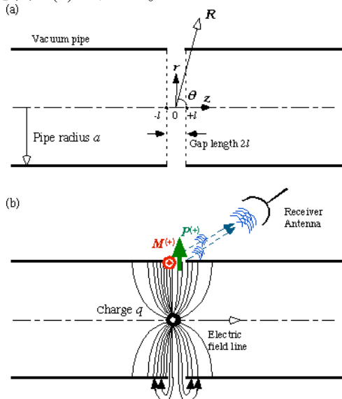
図1 : (a) 真空パイプとギャップの幾何学的大きさ、(b) 荷電粒子がギャップを通過するときの干渉性電磁放射の模式図
