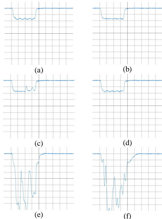
図3 狭導波管試験時に収集したブレイクダウン直前の反射波形
