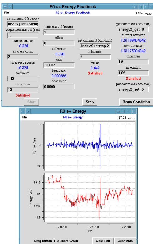
図 2: フィードバックの例として、R セクタのエネルギーフィードバックの設定パネルとグラフ。運転時であってもフィードバックの設定パラメータは簡単な前処理、後処理を含めて変更可能で、また、ソフトウェアのほとんどの部分は他のフィードバックと共通となっている。
