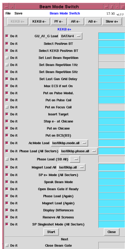
図 1: ビームモードスイッチパネルで、KEKB e^+ が指定した状態。左の Check-button で項目の選択、非選択を変更でき、また Pull-down menu でパラメータファイルを選ぶことができる。右端は実行状態を表す。
